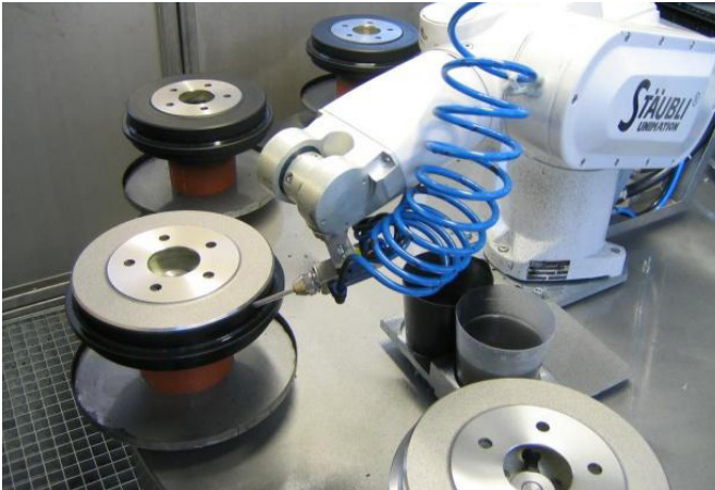
Rundautomat mit stabiler Teileaufnahme zur präzisen Beschichtung
